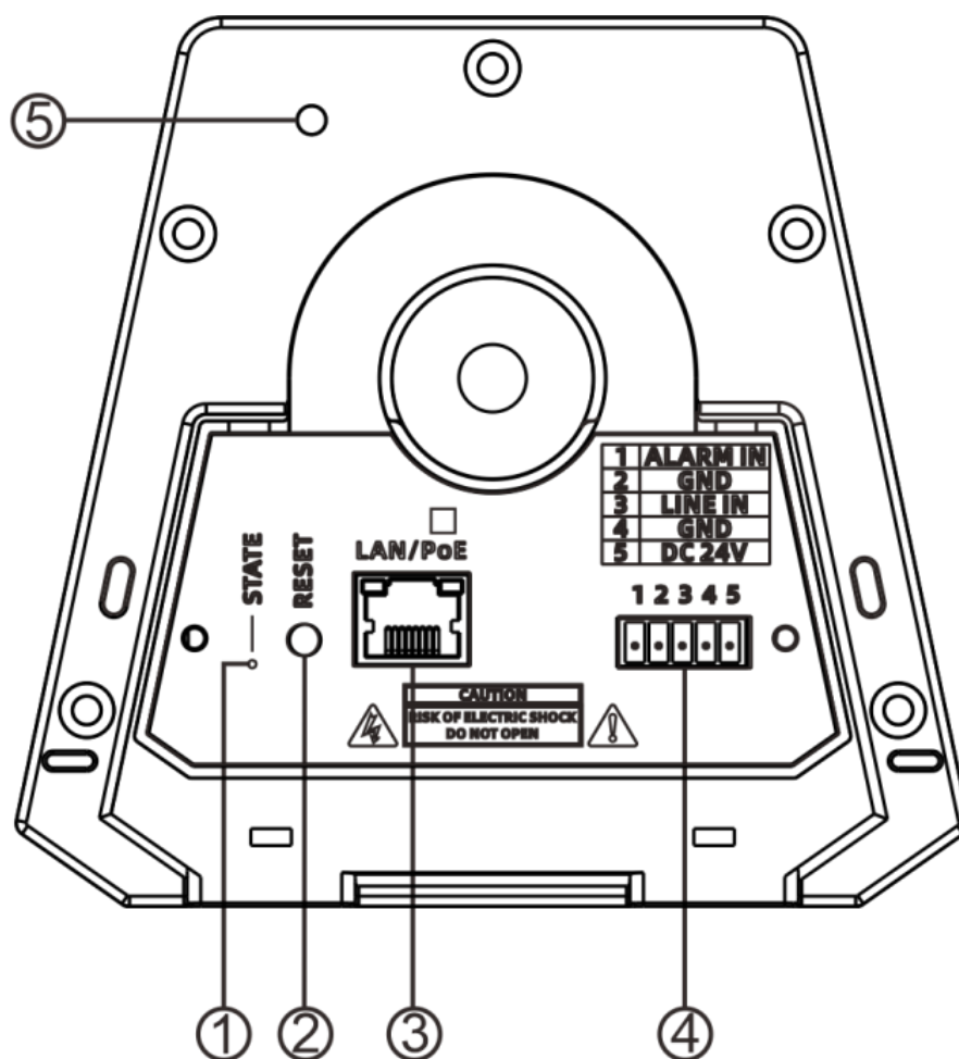
Рис. 2. Интерфейсы уличной IP-звуковой колонны LPA-6191A06
